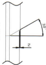
矢視A
